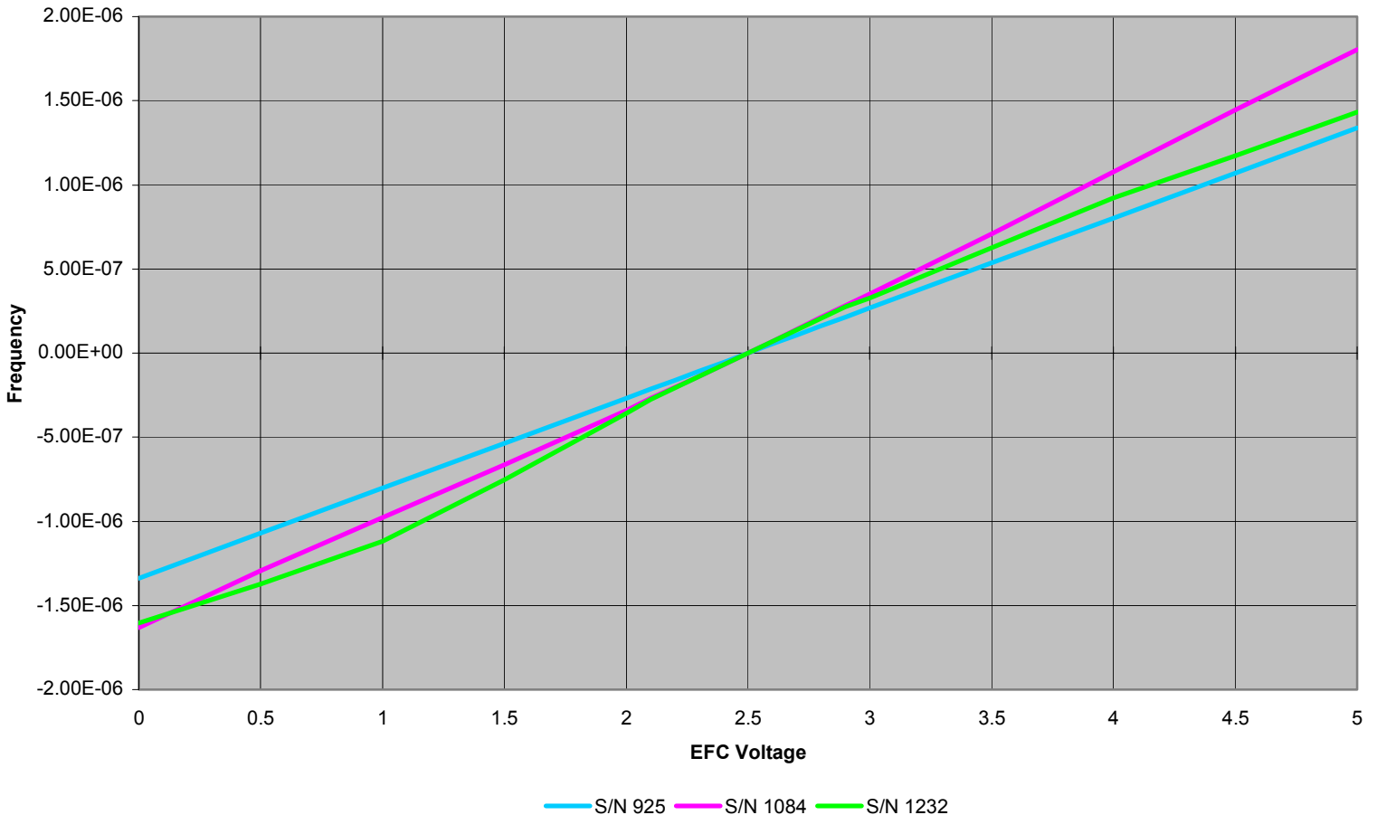
Mini Wonder EFC vs Frequency
